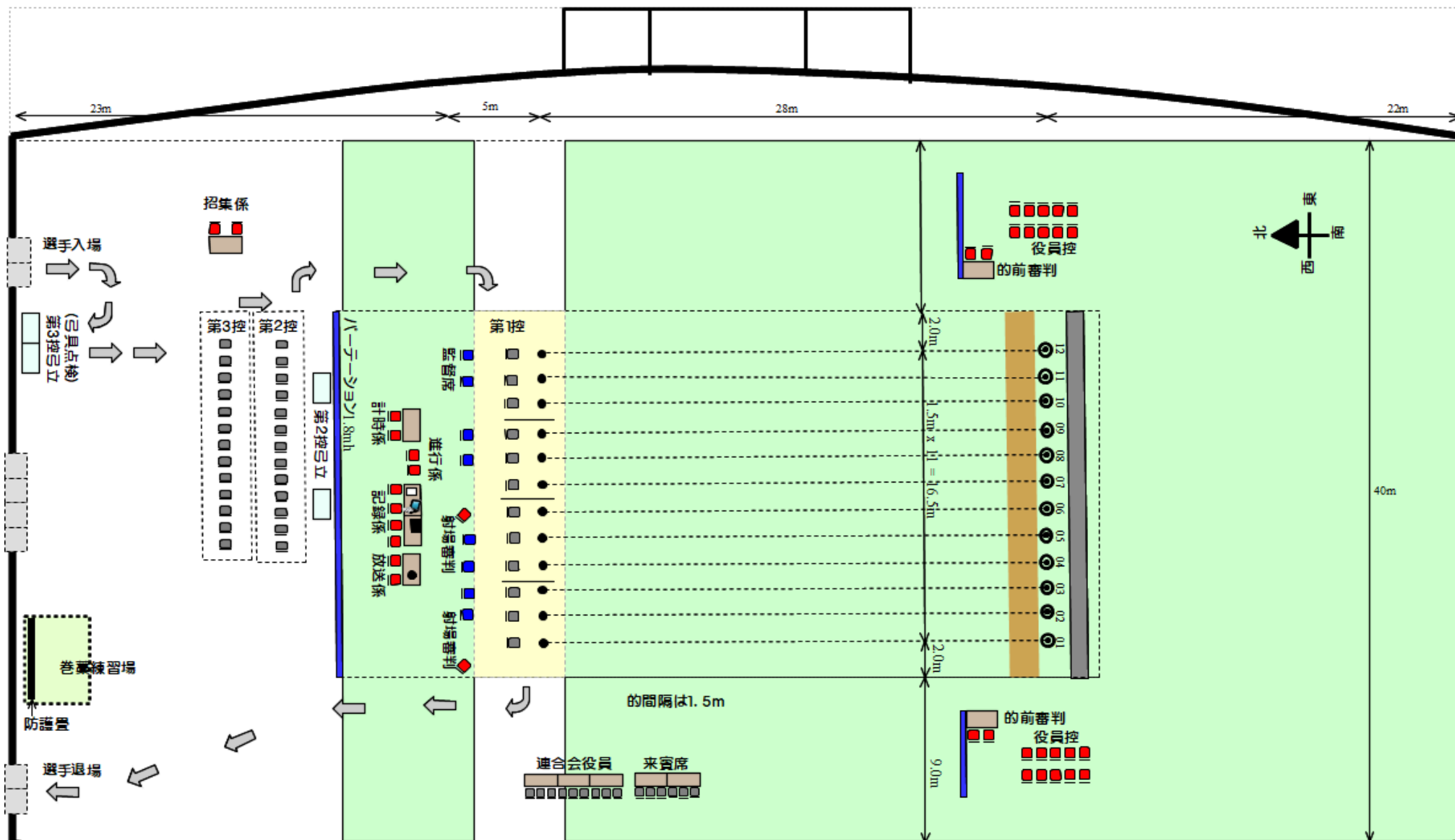
1F競技場レイアウト
